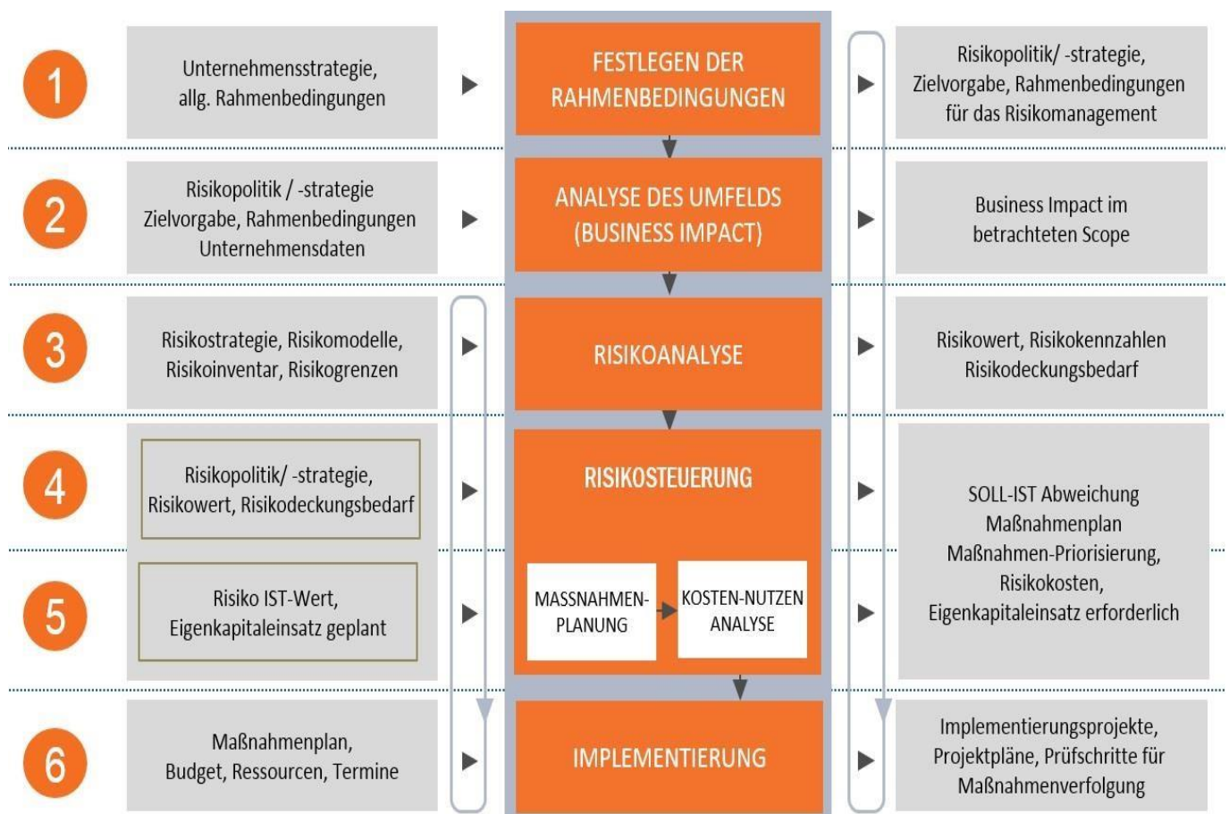
Abbildung 1: Prozess Informationssicherheit-Risikomanagement
